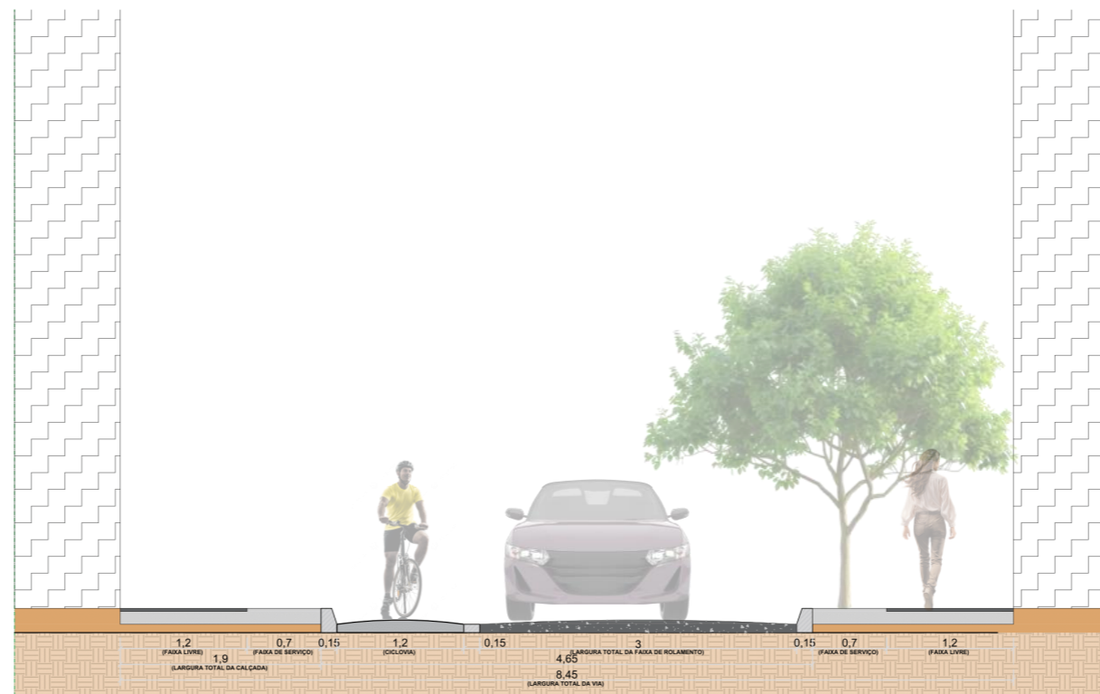
VIA COMPLETA - LOCAL
