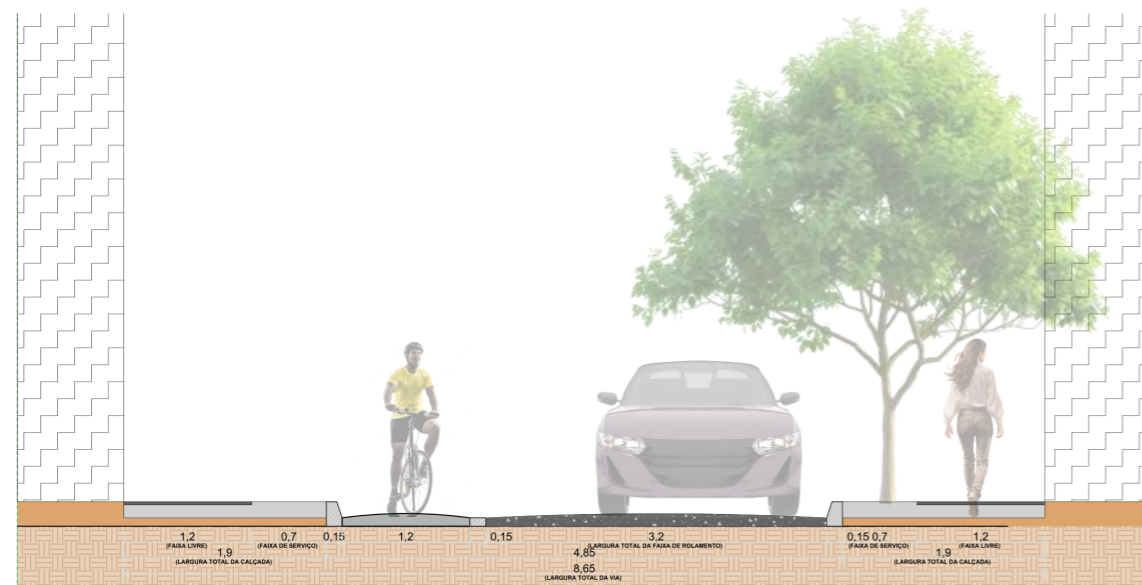
VIA COMPLETA - COLETORA
