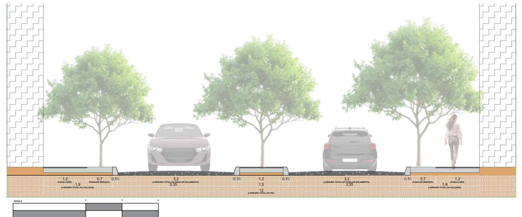
VIA COLETORA - MÃO DUPLA COM CANTEIRO
