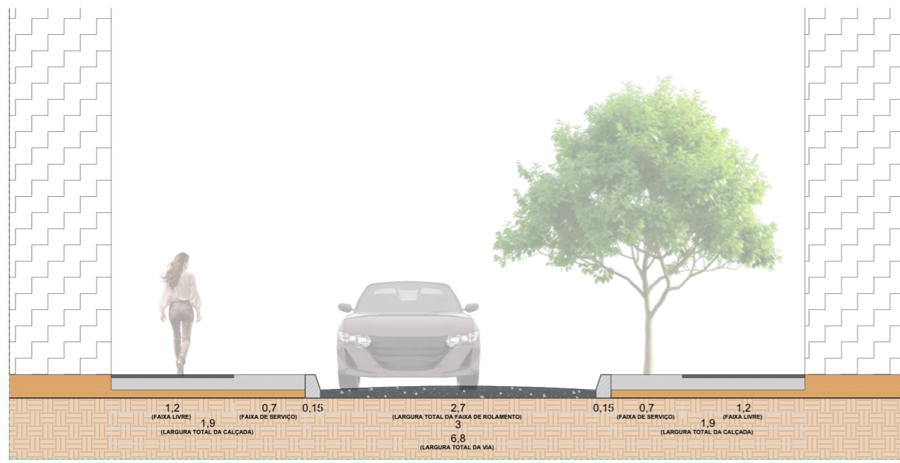
VIA LOCAL - ZEIS
