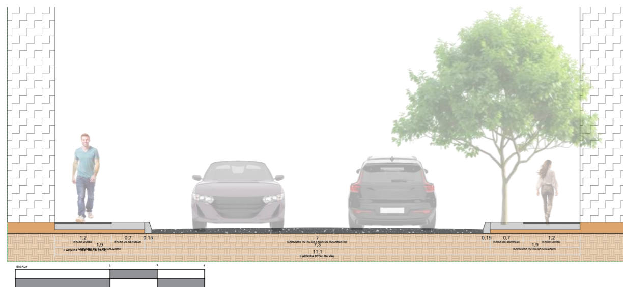
VIA ARTERIAL - MÃO DUPLA
