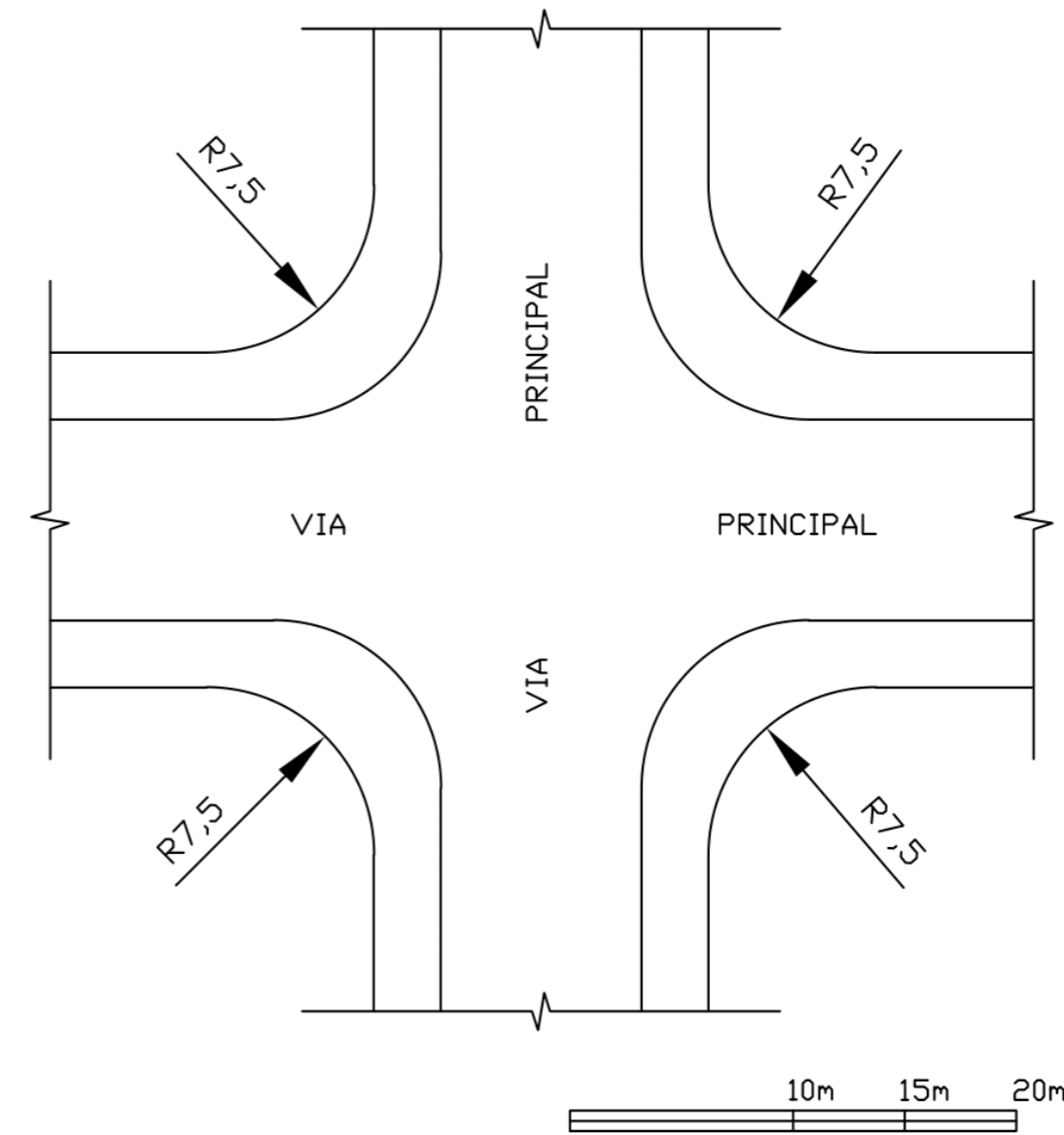
CUZAMENTO COLETORA COLETORA X COLETORA
